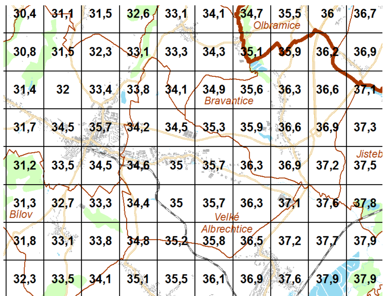
Obrázek 1-8: Koncentrace prachu PM10 ( \mu\text{g}/\text{m}^3 ) v obci a okolí – max. průměr za 24 hod
