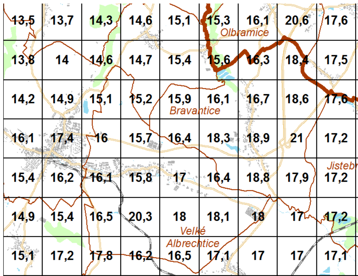
Obrázek 1-7 Roční průměr koncentrace oxidu dusičitého v obci a okolí: roční průměr ( \mu\text{g}/\text{m}^3 )
