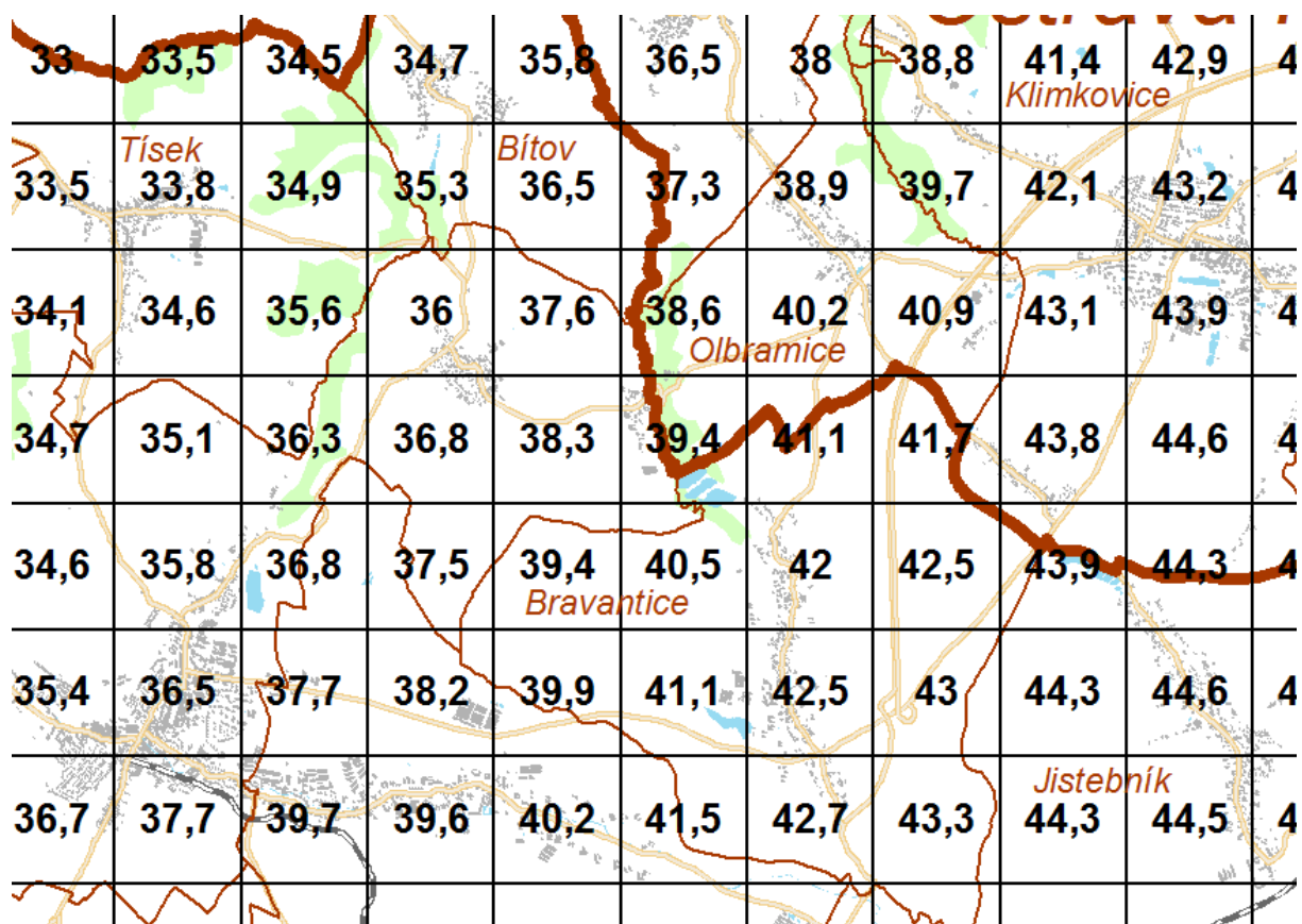
Obrázek 1-6 Koncentrace oxidu siřičitého v obci a okolí ( \mu\text{g}/\text{m}^3 max. koncentrace za 24 hodin)
